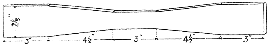
FIG. 1. TENSILE TEST SPECIMEN.
